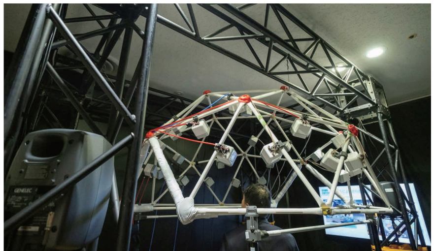
図3 ドーム型ノイズキャンセリング装置
