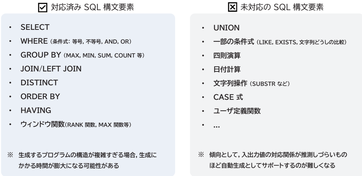
図1 自動生成できるSQLクエリの構文要素
